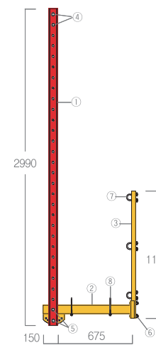
SFP-W75300A Platform framework components 平台框架组件
